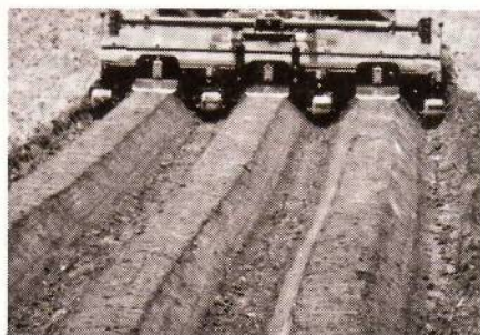
三畦成形機の作業状態
