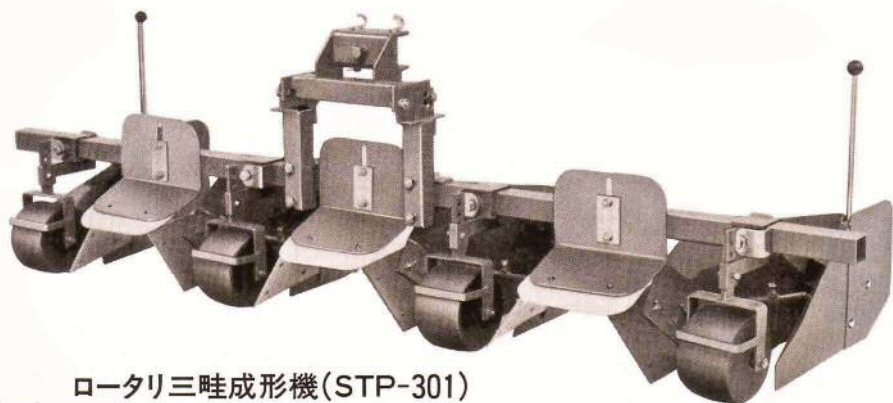
フロントゲージロータリ用 三畦成形機の例
